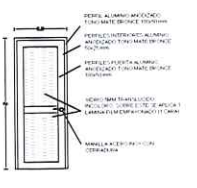
ELEVACION PUERTA TIPO ALUMBRADO VODAS
