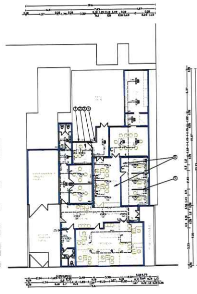
PLANTA HABITACION ETAPA #3 DISEÑO, MEJORAMIENTO DE ESPACIO RECIBIENDO INFORMACION ELECTRICA, ALUMBRADO Y RED DE VODAS DE DATOS.
